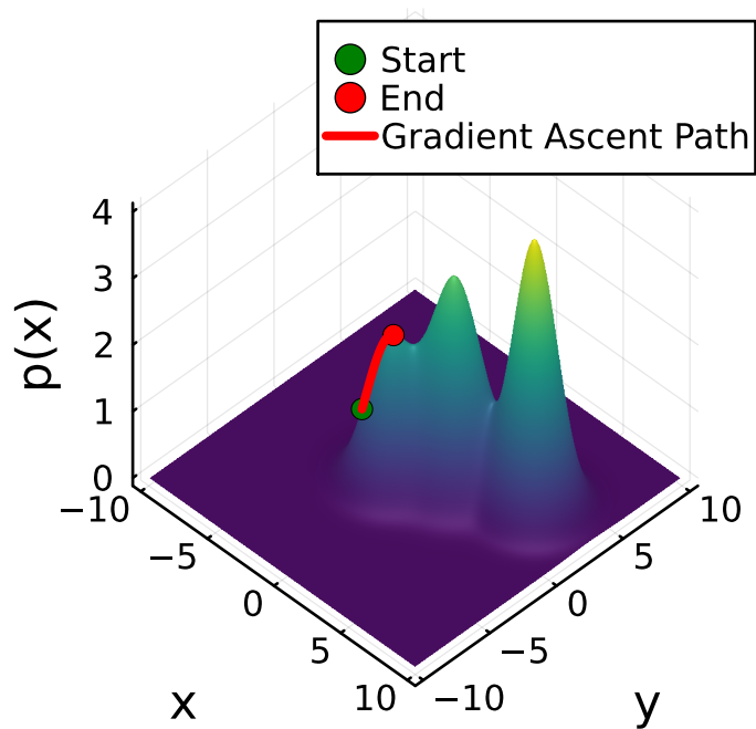
Gradient Ascent
